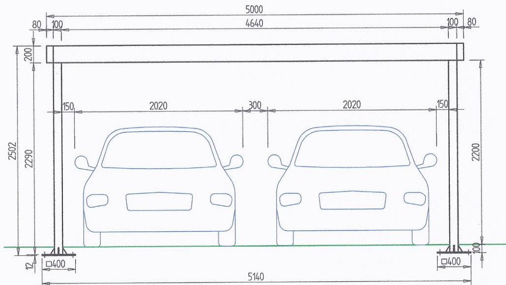
ČELNÝ POHLAD
