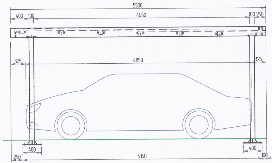
BOČNÝ POHLAD
