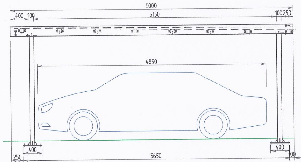
BOČNÝ POHLAD
