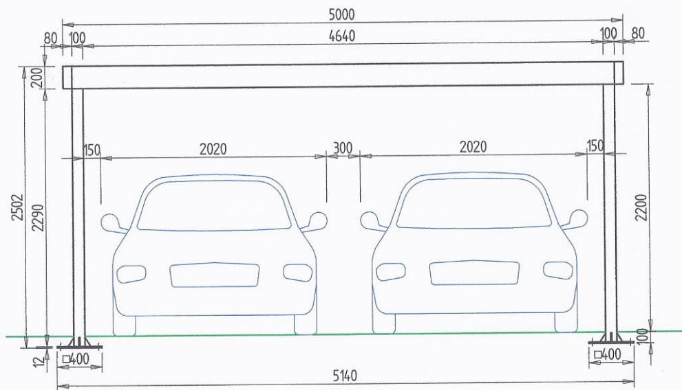
ČELNÝ POHLAD
