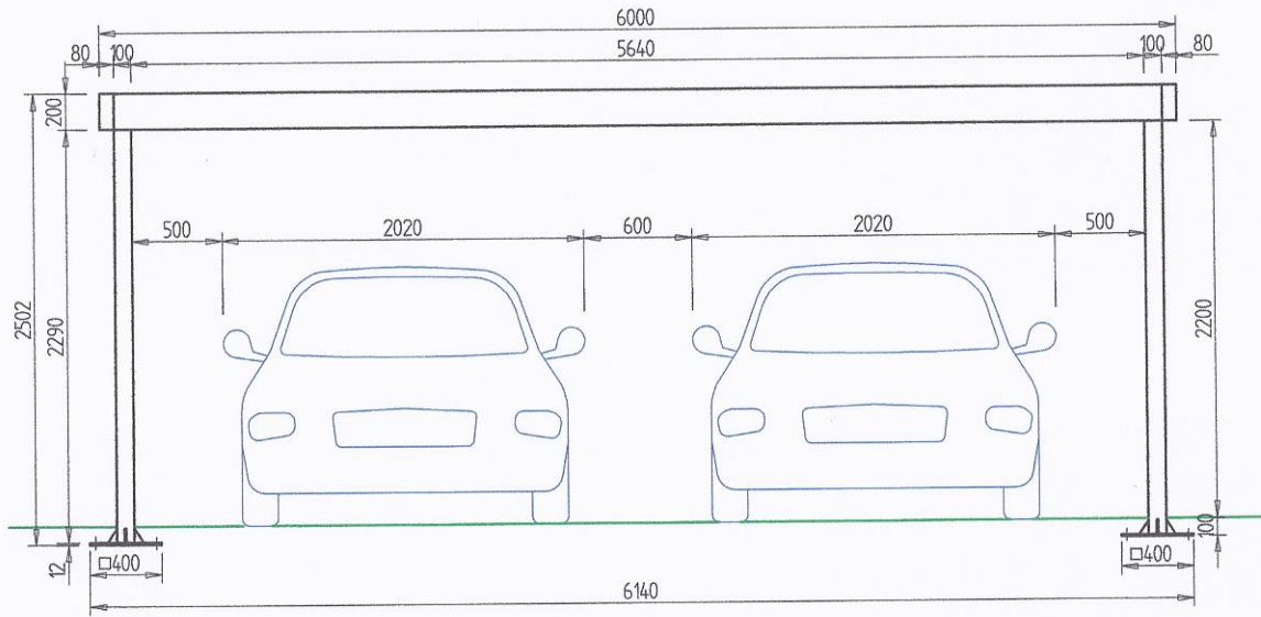
ČELNÝ POHLAD
