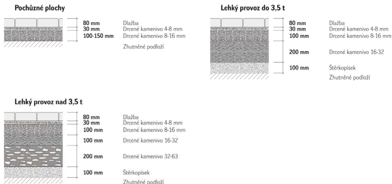
Obrázek č.2: Varianty skladeb při pokládce skladebné dlažby Brož Lucca® tl. 80 mm
