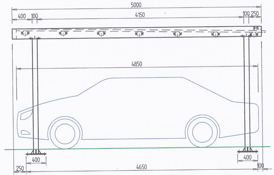
BOČNÝ POHLAD
