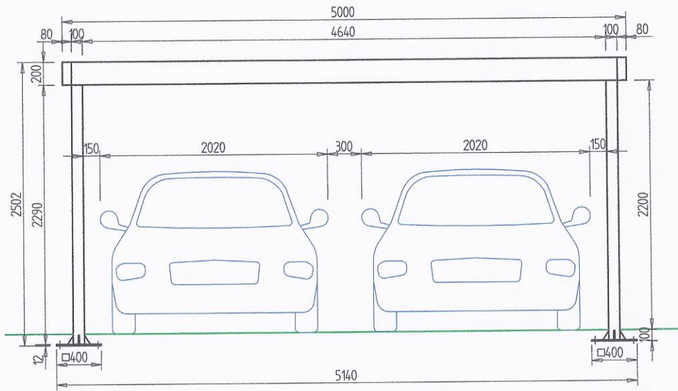
ČELNÝ POHLAD
