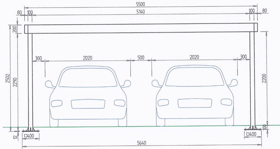
ČELNÝ POHLAD
