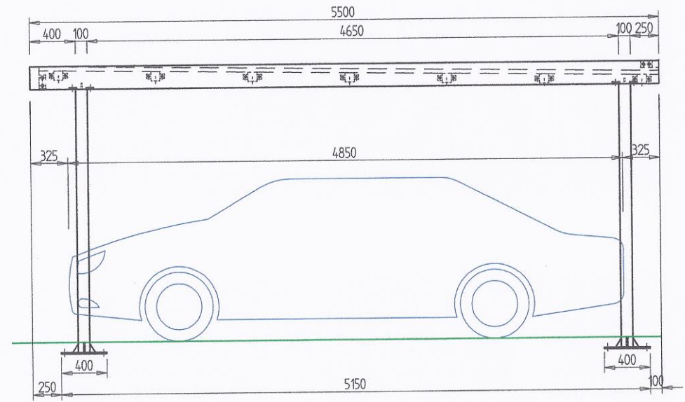
BOČNÝ POHLAD
