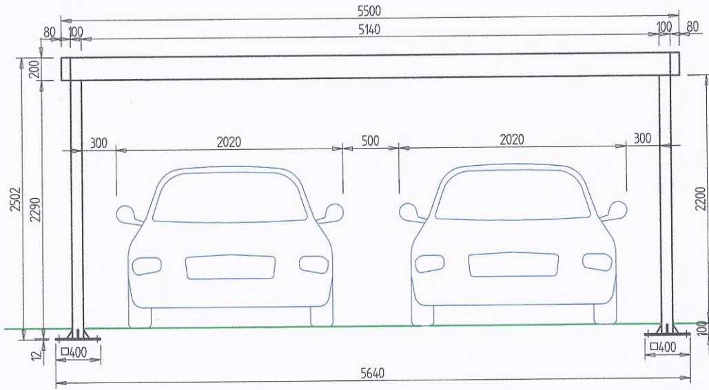
ČELNÝ POHLAD
