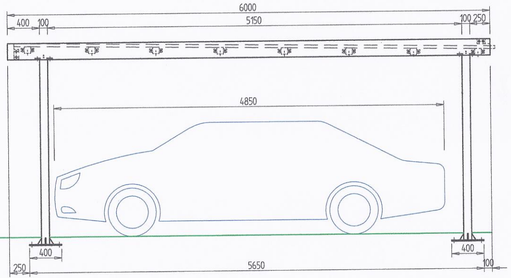
BOČNÝ POHLAD
