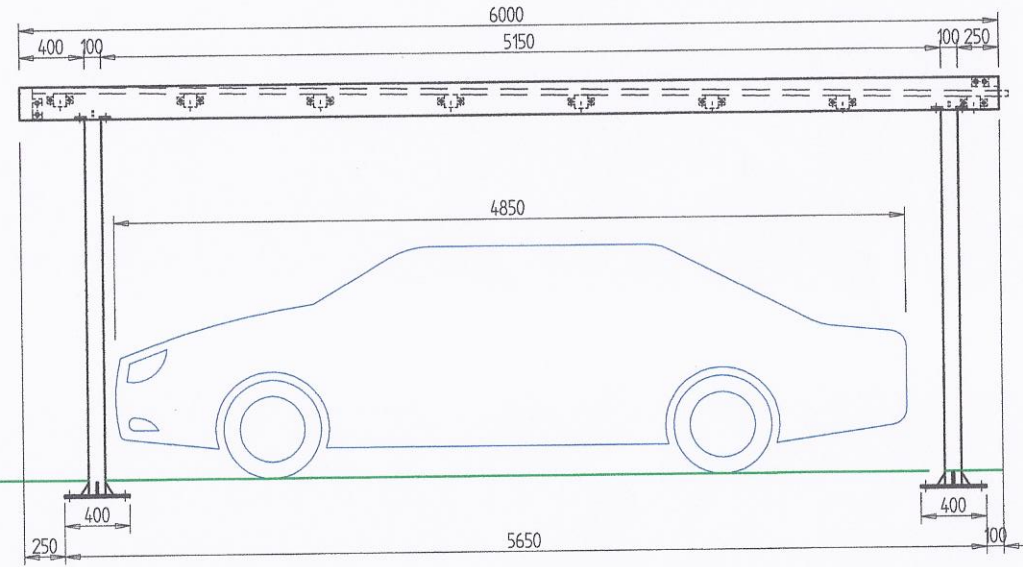
BOČNÝ POHLAD
