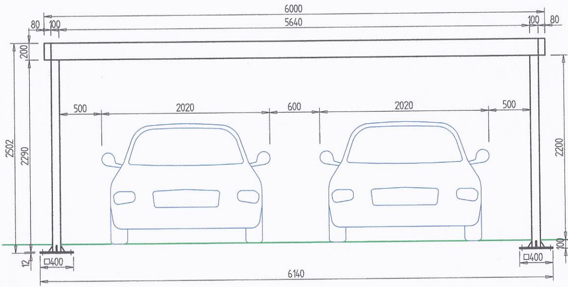
ČELNÝ POHLAD
