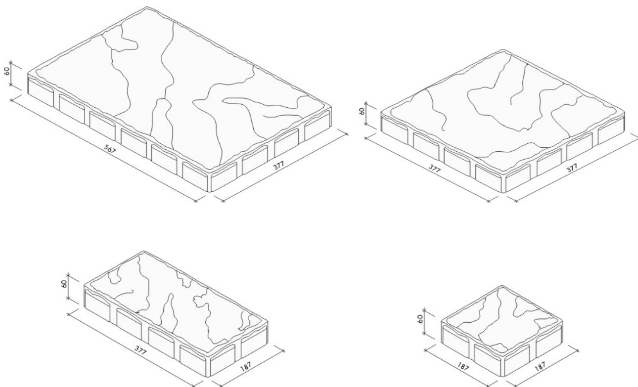
Obrázky č.1: Rozměrové parametry prvků
