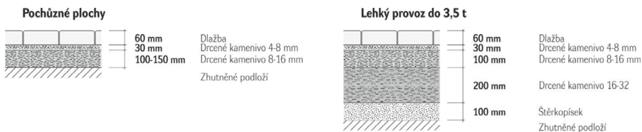
Obrázek č.2: Varianty skladeb při pokládce skladebné dlažby Brož Provance®, tl. 60 mm
