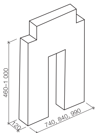
Zadní opěrná deska
