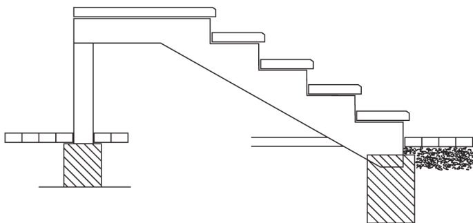
Usazení schodišťového systému do terénu
