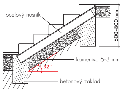
Uložení na ocelový nosník.
