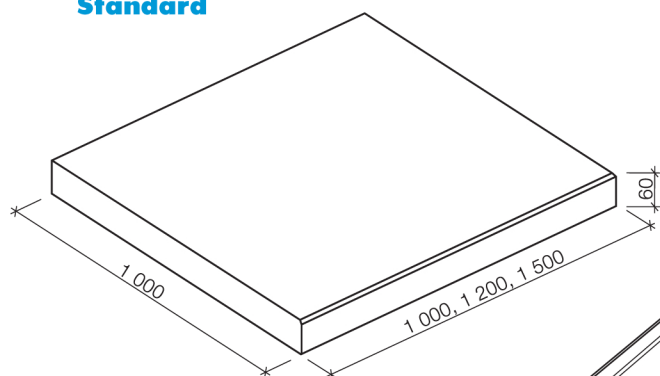
Podestová deska v provedení Standard
