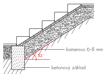
Uložení do šterkového lože: pro menší, jednoduché, v terénu volně osazená schodiště.
