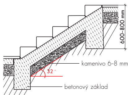
Uložení na betonový základ: pro dlouhá nebo široká schodiště, pro schodiště připojená k budovám a zídám.
