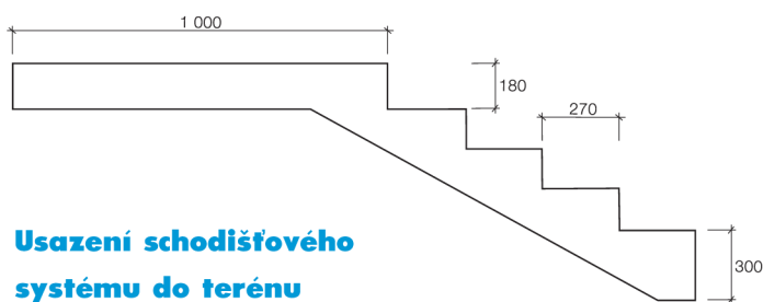
Schodišťové rameno – 5 stupňů
