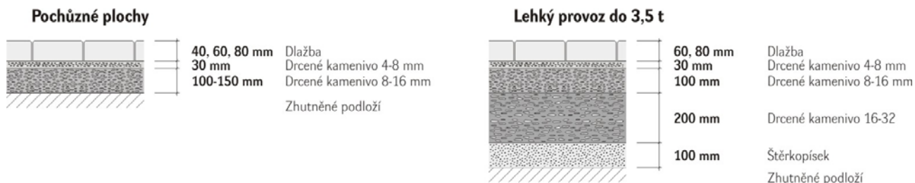
Obrázek č.2: Varianty skladeb při pokládce skladebné dlažby Brož Valletta® , tl. 60 mm
