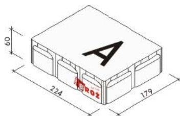
Obrázky č.1: Rozměrové parametry prvků
